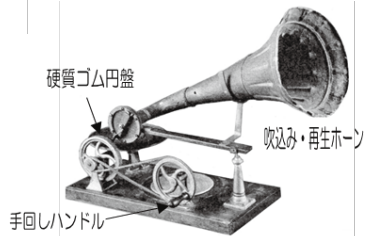
図2 発明時のベルリナー式
