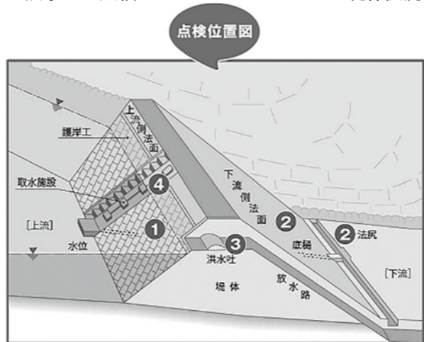
▲堤体法尻の点検
