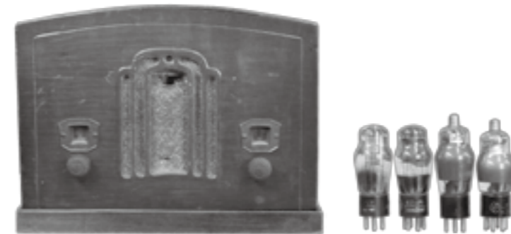
大きさ:24cm(高さ)、34cm(幅)、20cm(奥行き)、5kg(重さ) 使用されているST型真空管
