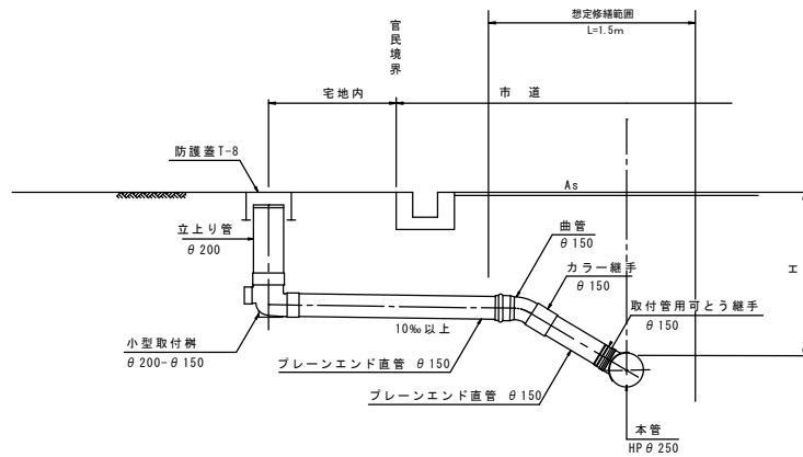
取付管布設断面図
