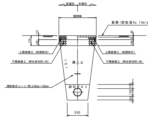
復旧断面図(市道)
