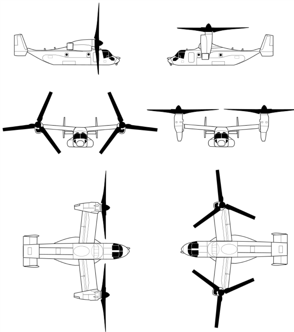
MV-22 三面図 右が垂直離着陸モード，左が固定翼モード 出典 フリー百科事典「ウィキペディア」
