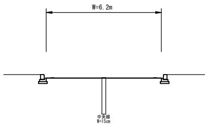
標準横断面図 S=1:100
