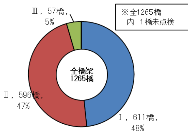
図1-5 定期点検結果に基づく健全性
