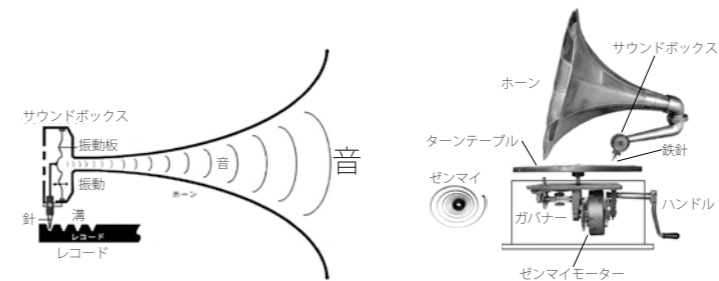
図-3 蓄音機の原理-2 図-4 蓄音機の仕組み
