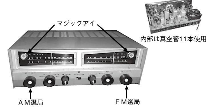
内部は真空管11本使用 大きさ：13cm(高さ)、38.5cm(幅)、21cm(奥行き)・重さ：5.7kg
